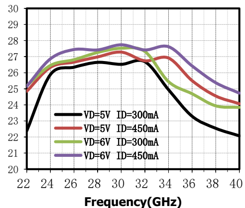
OP 1 dB(dBm) vs. V_D , I_D
