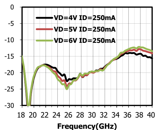
Output Return Loss(dB) vs.Bias
