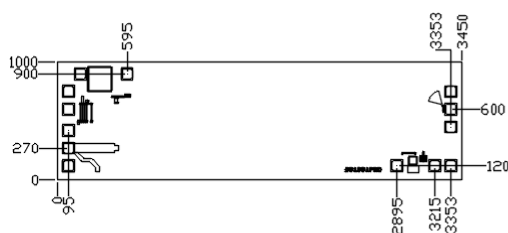
Die Outline (μm)
